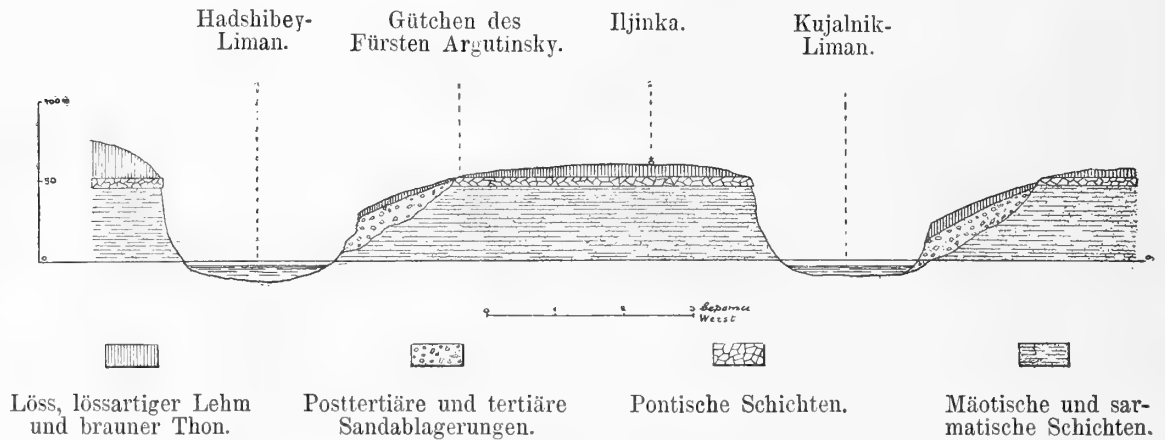
Geologischer Durchschnitt vom Dorfe Woljanowka (an der Westküste des Hadshibey-Limans) über Iljinka bis Kubanka (an der Ostküste des Kujalnik-Limans) 1) .
